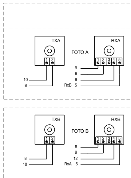
fig. 4b Foto A e foto B con collegamento per fototest
