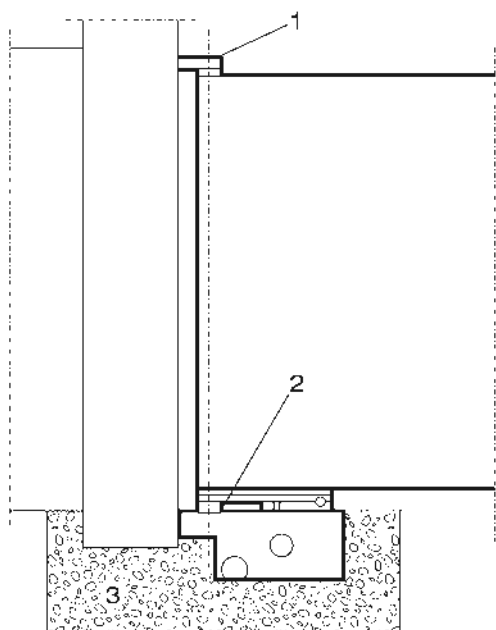
1- Stützzapfen 2- Zapfen 3- Stahlbeton
