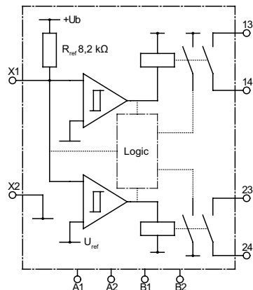
Prinzipialschaltbild SK 41
