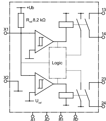
Prinzipschaltbild SK 41
