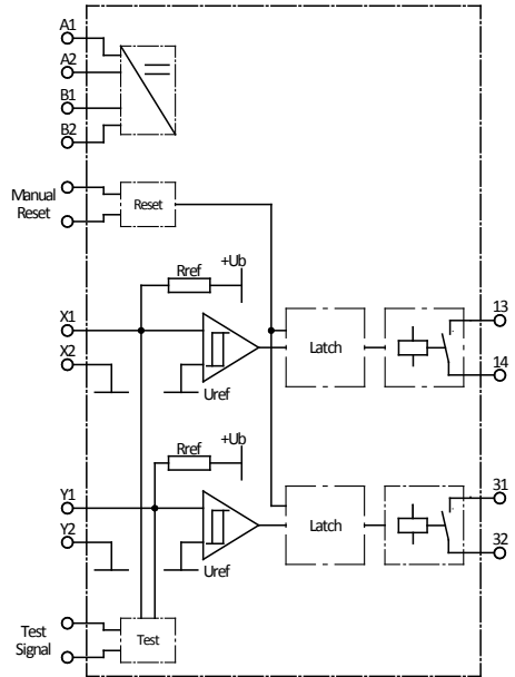
Prinzipschaltbild SK 35
