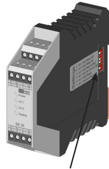
Commutateurs DIP
