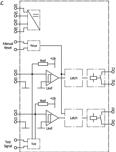
Principeschema SK 35
