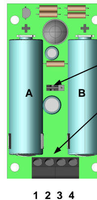
J2: Selección alimentación J1: Terminales para el contacto del borde sensible
